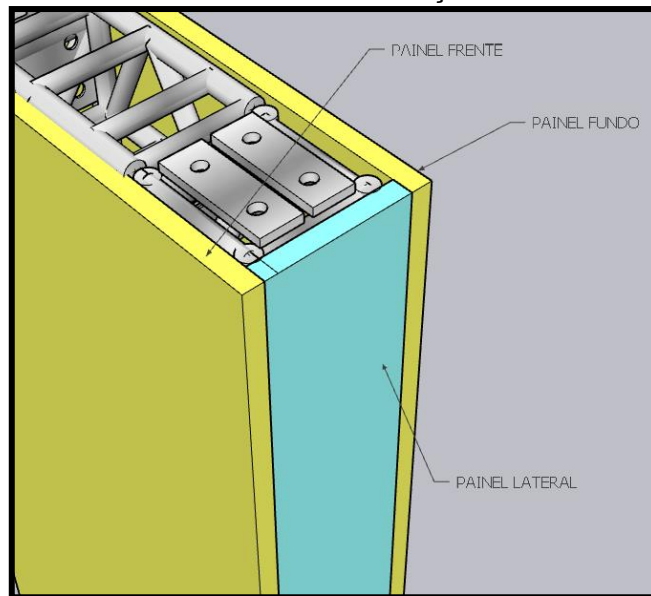
FIGURA 4: DETALHE DE INSTALAÇÃO DOS PAINÉIS
