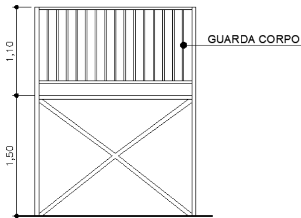
FIGURA 6: TORRE DE APOIO (CORTE)
