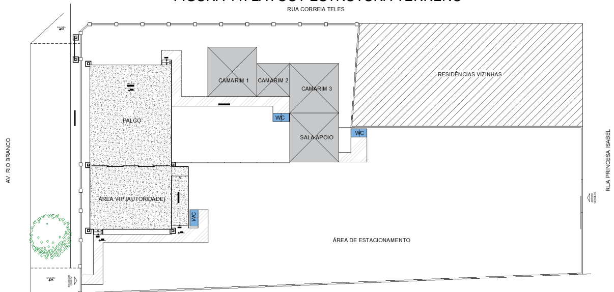
FIGURA 11: LAYOUT ESTRUTURA TERRENO
