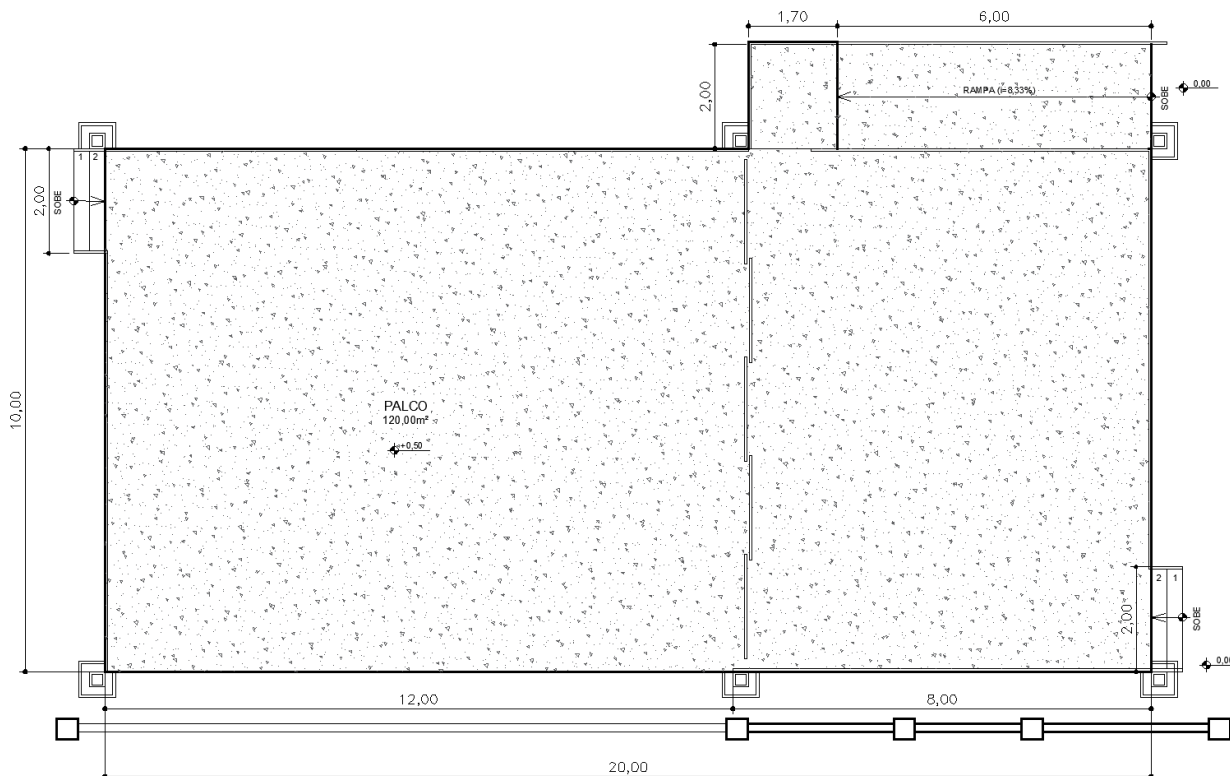
FIGURA 8: PALCO (CORTE ESQUEMÁTICO)
